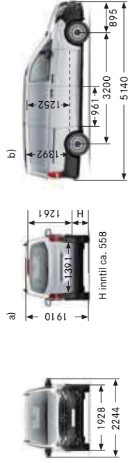
Varebil lang med 3200 mm akselavstånd
